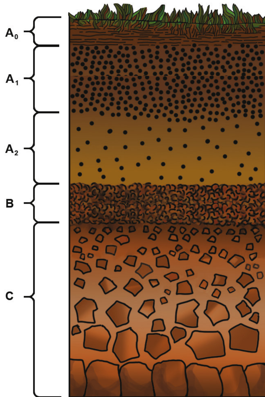
Dirvožemio profilis
